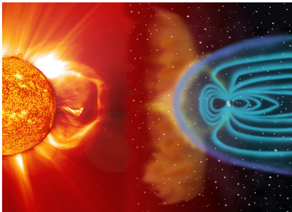
太阳风暴对地球的影响(电脑模拟图)
